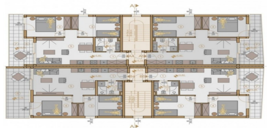
MJ 1:100
